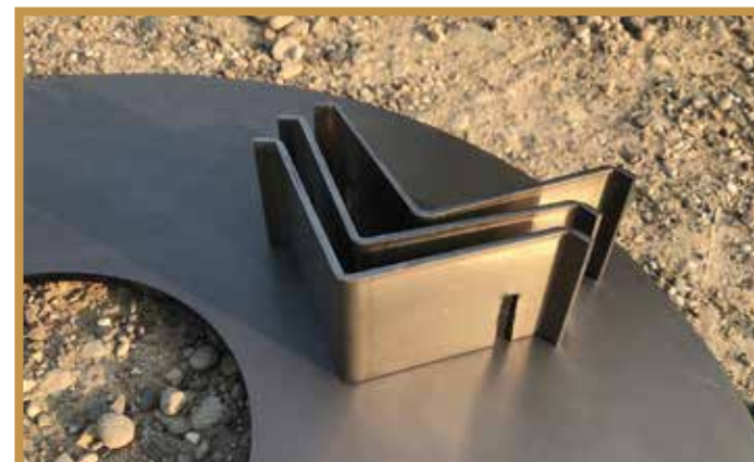
Grillplatten-/Grillrosthälter Edelstahl
