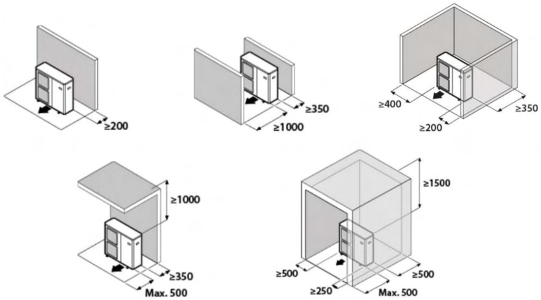
Mindestabstände für den Einbau eines Gerätes (mm).
