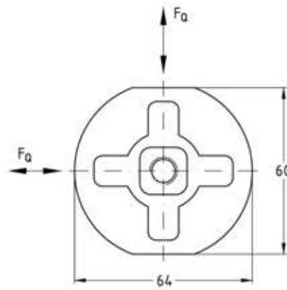
Schallentkoppelte Deckenbefestigung
