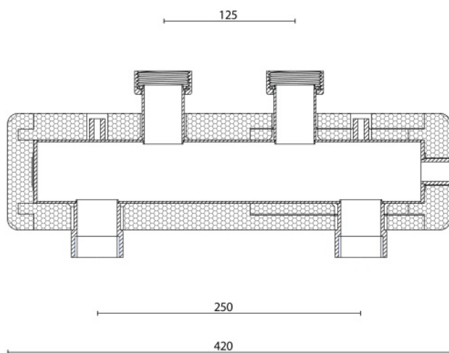
QUERSCHNITT
