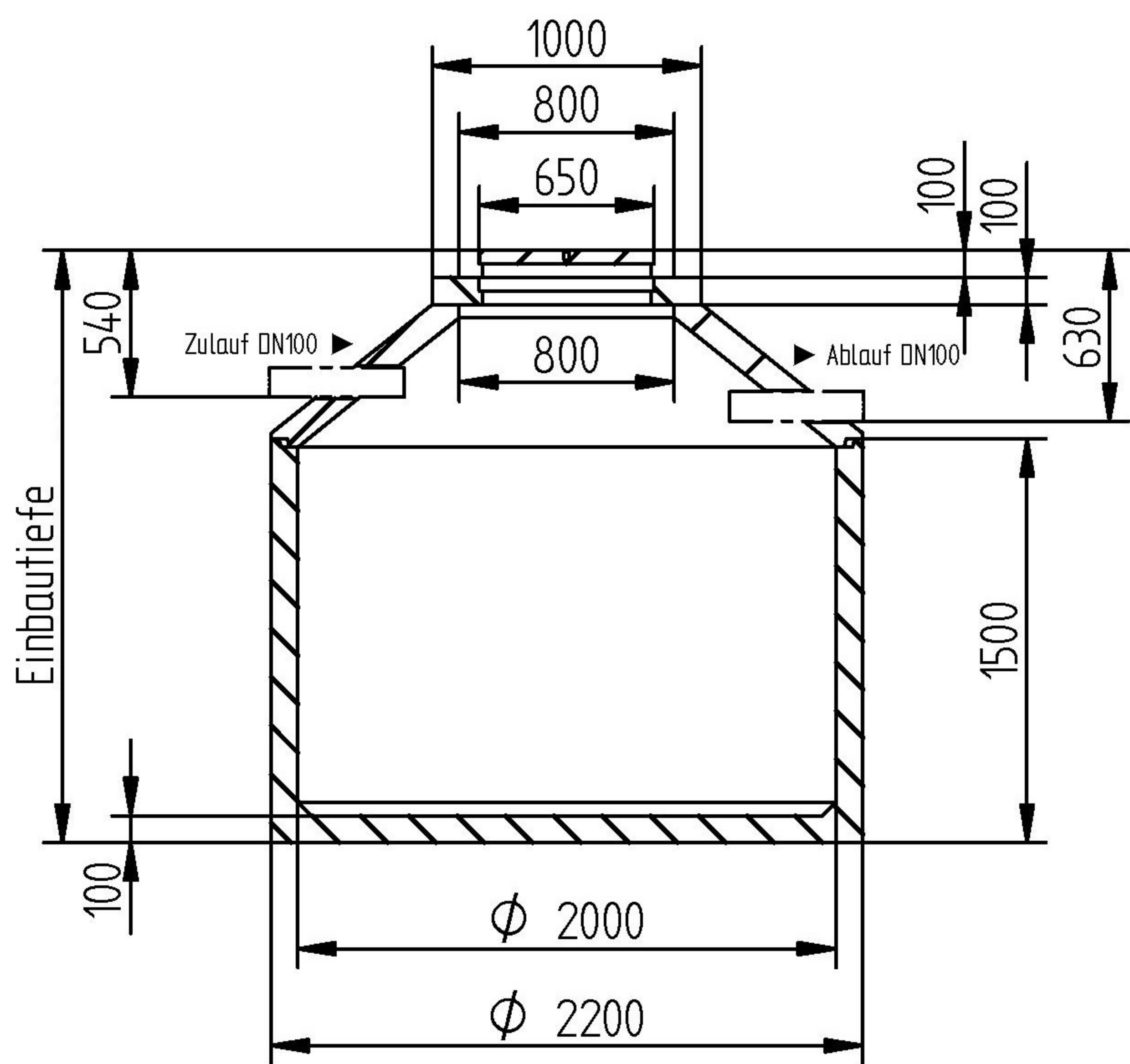
Schnitt A-A
