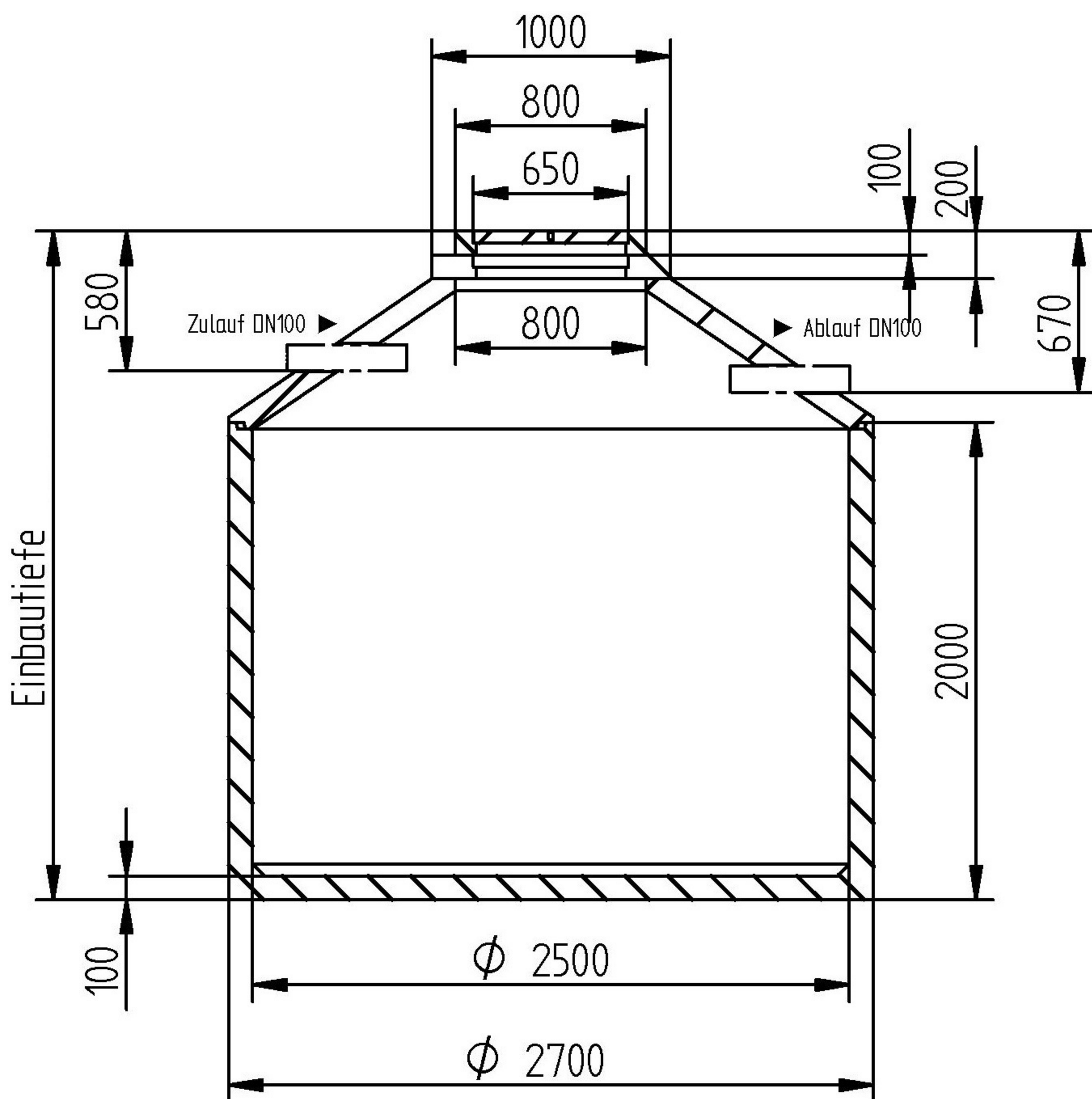
Schnitt A-A
