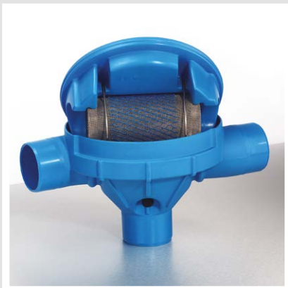
3P Sinusfilter 0 cm Höhenversatz
