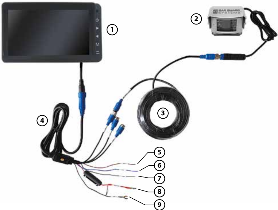
Abb. 3: Installation bei nicht serienmäßig vorinstalliertem Kamerakabel
