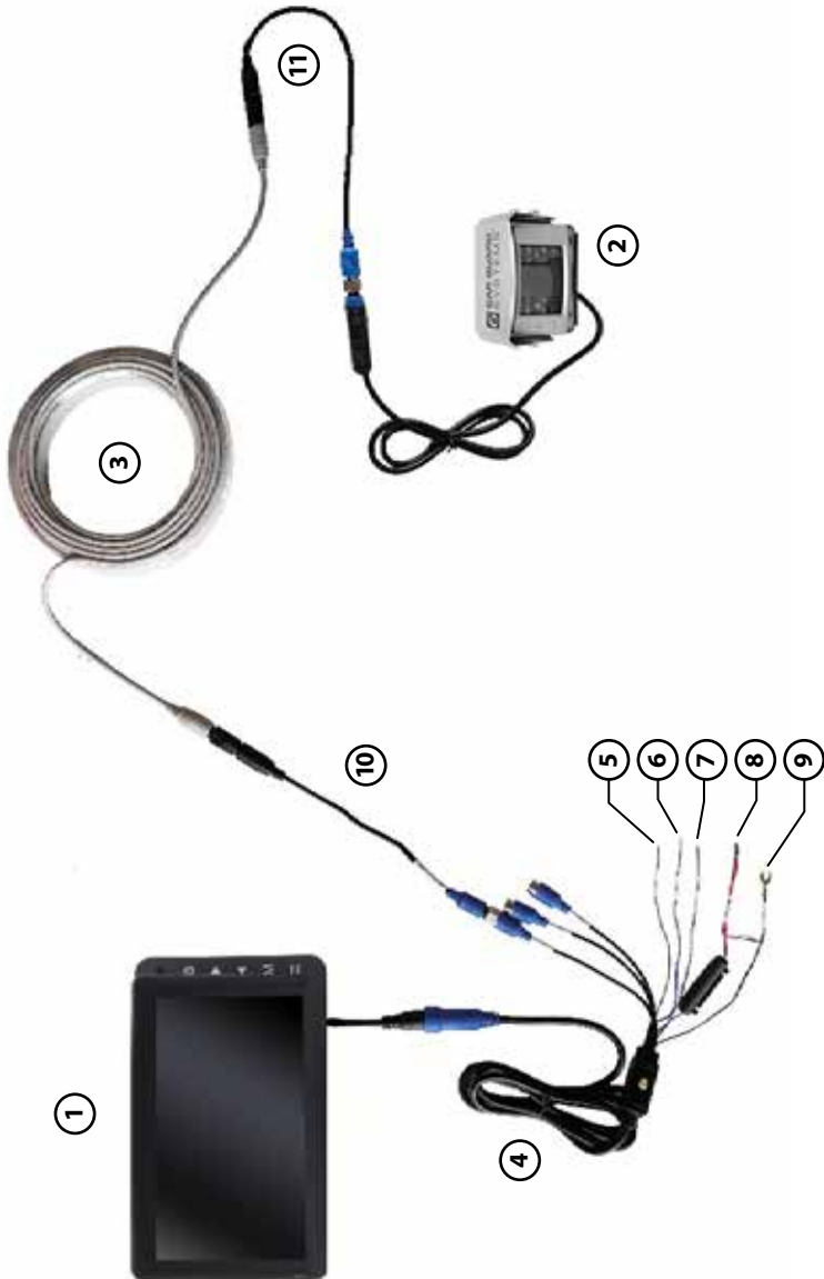
Abb. 4: Installation bei serienmäßig vorinstalliertem Orloco-Kamerakabel
