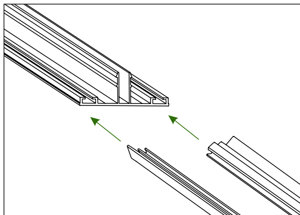
Sparrenabdeckprofile
