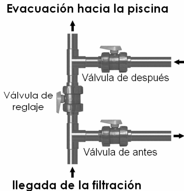
Esquema By-pass
