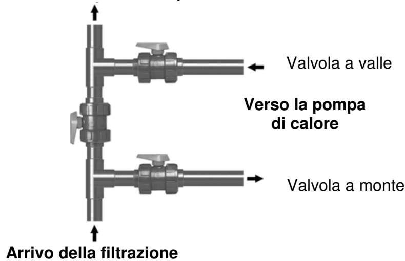
Schema del by-pass
