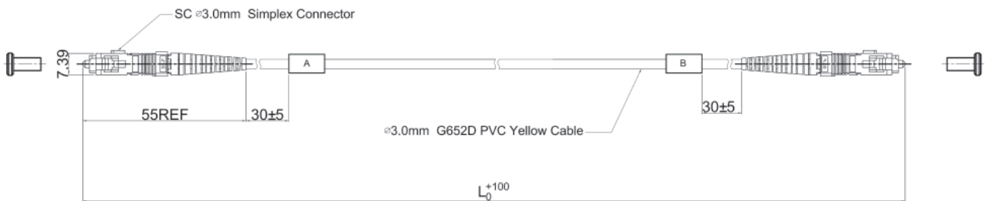
PCFAPC-S Serie - Abmessung in mm
