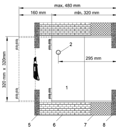
Ansicht von Seite / Einbaudarstellung NEUBAU
