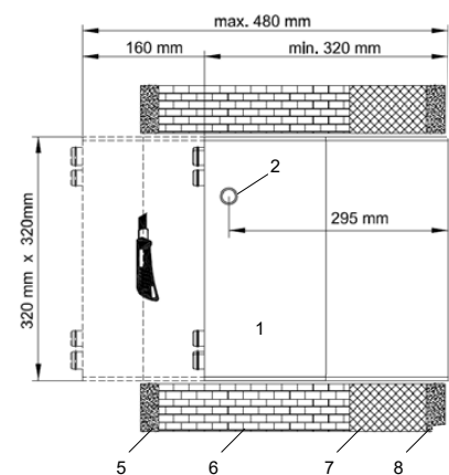
Ansicht von Seite / Einbaudarstellung SANIERUNG
