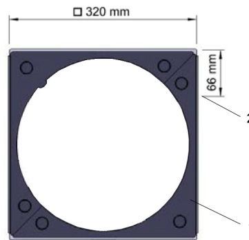
Ansicht von Raumseite
