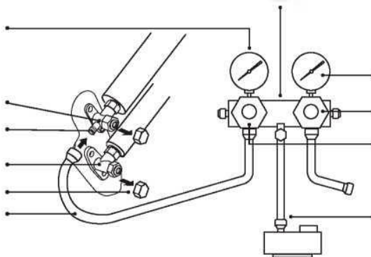
Vakuumpumpe
