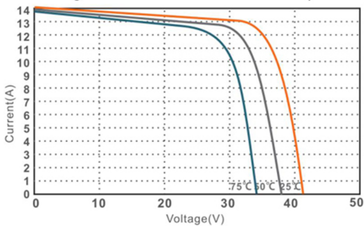
Leistungskennlinie bei verschiedenen Temperaturen
