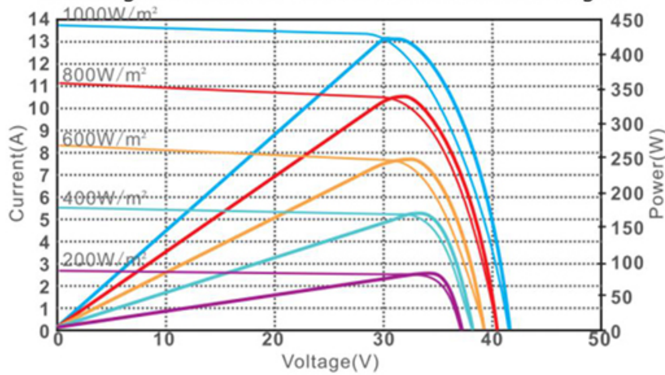
Leistungskennlinie bei verschiedenen Bestrahlungen
