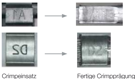
Crimpeinsatz
