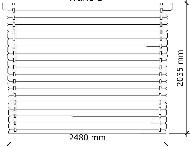
Wand B
