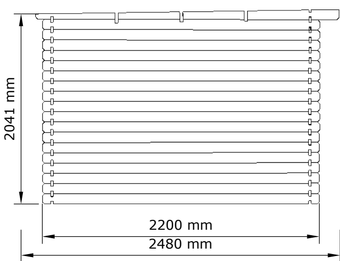
Wand C-D
