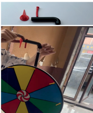
SCHRITT 7: Die Winkelstücke in der im Diagramm gezeigten Reihenfolge montieren und oben an der Halterung befestigen.
