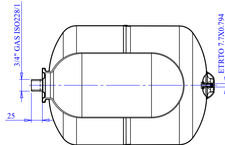
SEZIONE E-E
