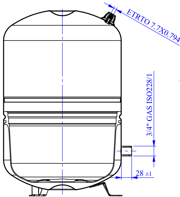
SEZIONE A-A
