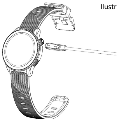
Podłącz inteligentny zegarek do kabla ładującego USB
